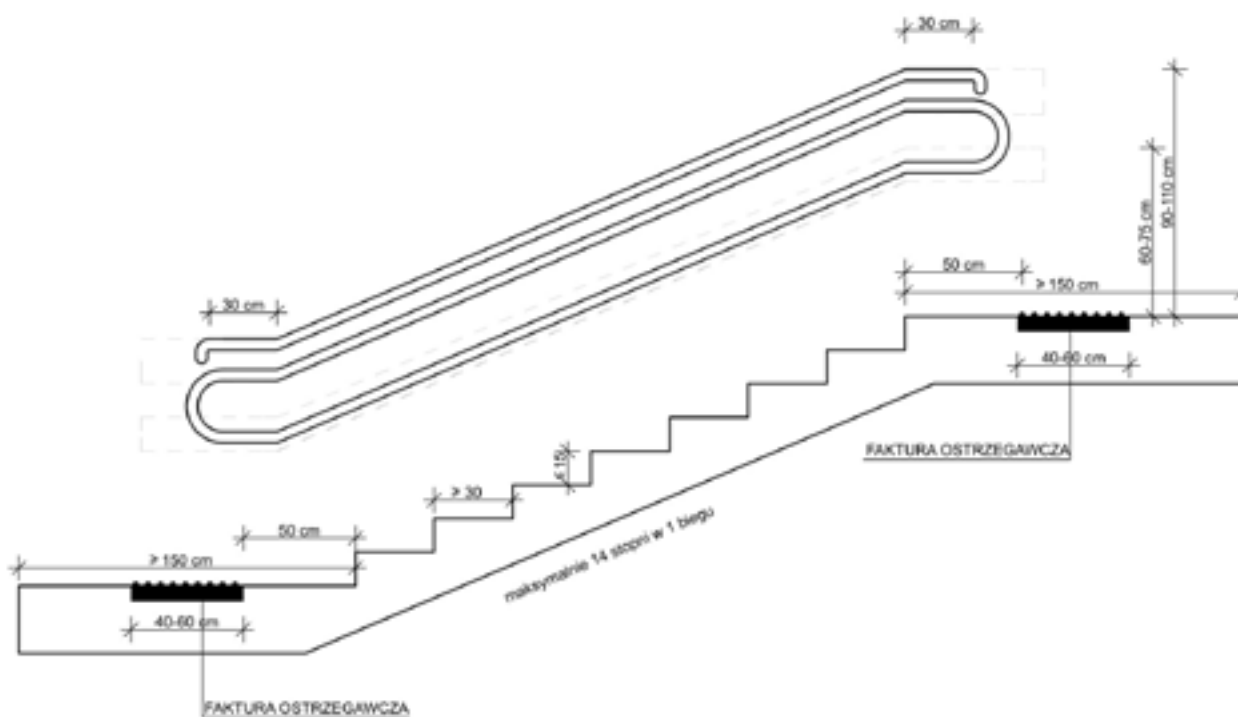
Schemat 5. Schody wewnętrzne Autor: Konrad Kowalczyk
