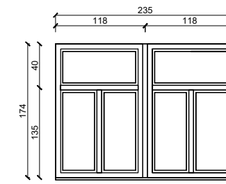
O1.5-1SZT STOLARKA O ODPORNOŚCI OGNIOWEJ EI60
