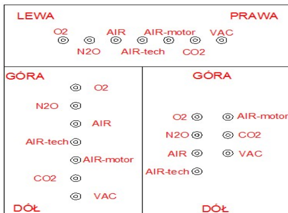
Rysunek 1 Sposoby montażu przewodów względem siebie
