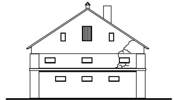
ELEWACJA POŁUDNIOWA
